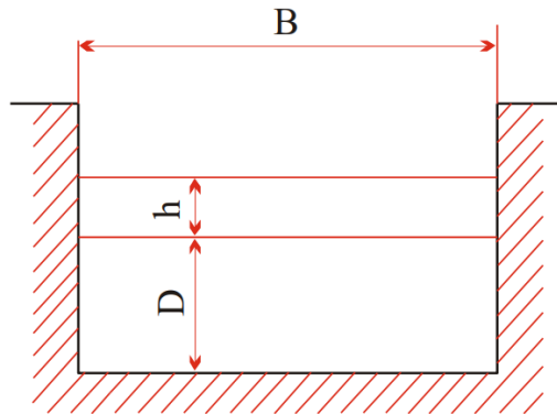
圖 12 全幅堰
